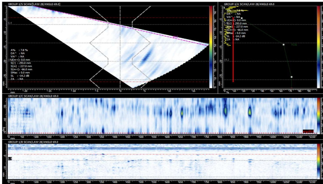
SPOOL-001 JUNTA-003
