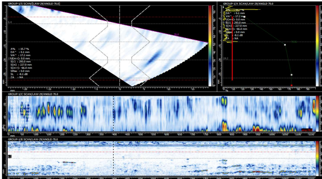
SPOOL-001 JUNTA-004
